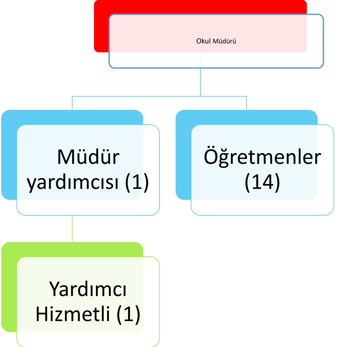
Şekil 8: Teşkilat Şeması
